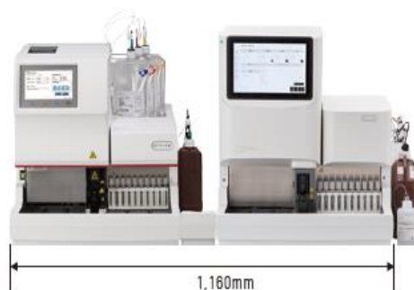
GA-1180とHA-8190Vの接続例
